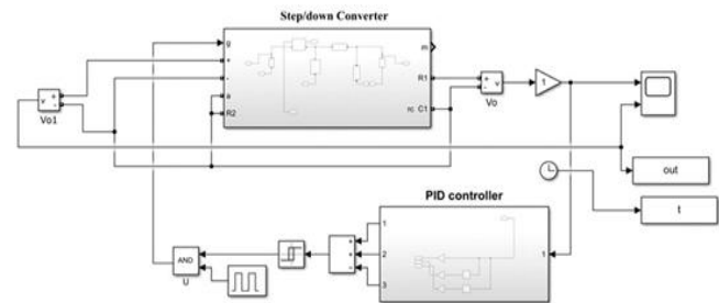
Fig. 6. PID using Z-N.
